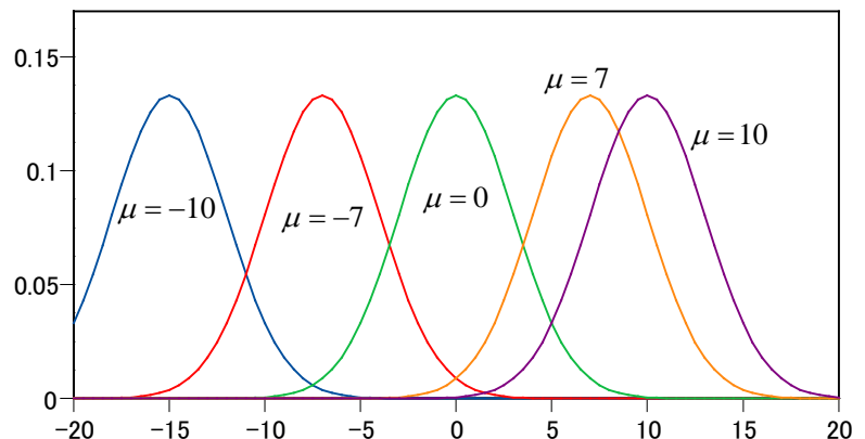
図-1 標準偏差を固定し、平均を変えたときの正規分布の確率密度関数
